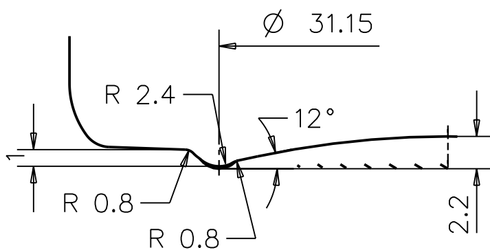
Pormenor do fundo de empilhar Esc.: 2/1
