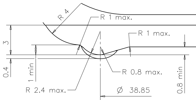
Pormenor do fundo Esc.:5/1
