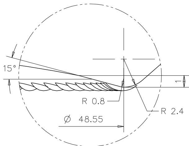
C Pormenor do fundo CarnaudMetalbox FD114 Esc. 5/1
